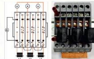
Короткозамыкающий штекер SCS 2-6 в разомкнутом состоянии
