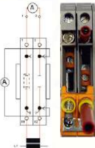
Сдвижная перемычка ZUK 2-6 T в разомкнутом состоянии
