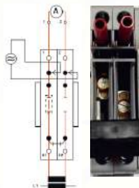
Короткозамыкающий штекер SCSS 2-6 в замкнутом состоянии
