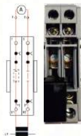
Короткозамыкающий штекер SCSS 2-6 в разомкнутом состоянии
