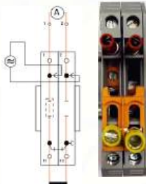
Сдвижная перемычка ZUK 2-6 T в замкнутом состоянии
