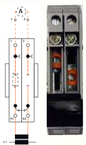
Короткозамыкающий штекер SCS 2-6 в замкнутом состоянии
