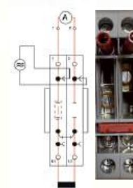
Ножевая перемычка ZUK 2-6 в замкнутом состоянии
