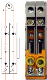
Сдвижная перемычка ZUK 2-6 T в разомкнутом состоянии
