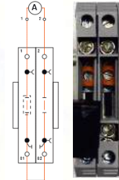
Короткозамыкающий штекер SCS 2-6 в разомкнутом состоянии
