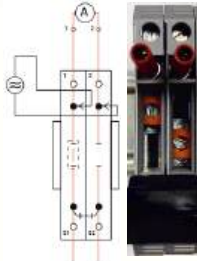
Короткозамыкающий штекер SCS 2-6 в замкнутом состоянии
