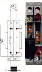
Короткозамыкающий штекер SCS 2-6 в разомкнутом состоянии
