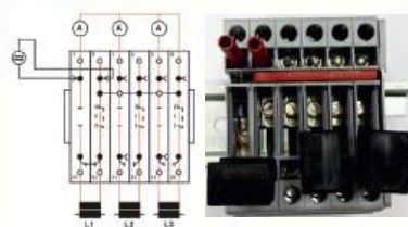
Короткозамыкающий штекер SCSS 2-6 в замкнутом состоянии
