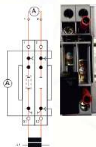
Короткозамыкающий штекер SCSS 2-6 в разомкнутом состоянии
