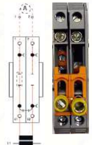
Сдвижная перемычка ZUK 2-6 T в замкнутом состоянии
