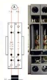
Ножевая перемычка ZUK 2-6 в разомкнутом состоянии
