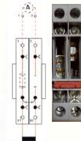
Ножевая перемычка ZUK 2-6 в замкнутом состоянии
