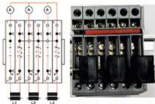
Короткозамыкающий штекер SCSS 2-6 в разомкнутом состоянии
